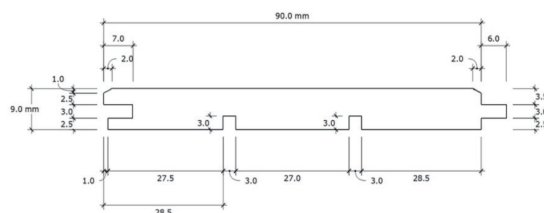
〈断面図〉
