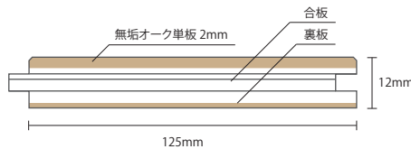
■ 断面図
