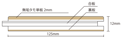
■ 断面図
